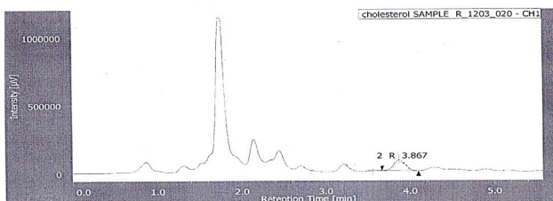
شكل 6: كروماتوجرام عينة لبن الأبقار
