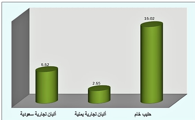
شكل 15: مقارنة بين متوسط محتوى الكوليسترول في الألبان اليمنية والسعودية mg/100g بيانياً
