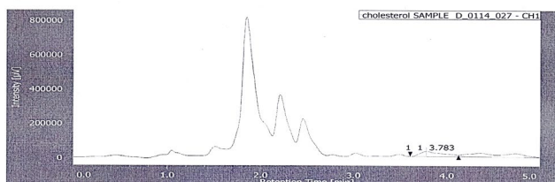
شكل 9: كروماتوجرام عينة مراعي كامل الدسم
