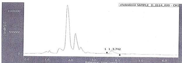
شكل 4: كروماتوجرام عينة لبن ضأن
