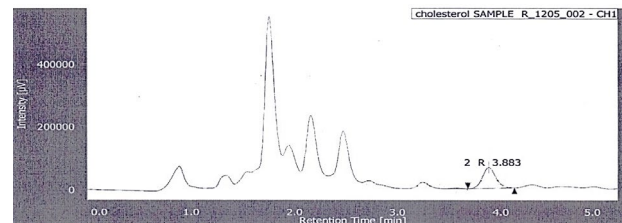
شكل 7: كروماتوجرام عينة ندى كامل الدسم
