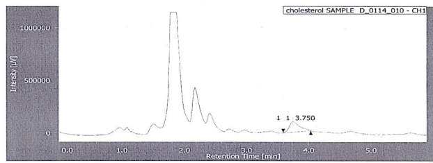
شكل 3: كروماتوجرام عينة لبن ماعز
