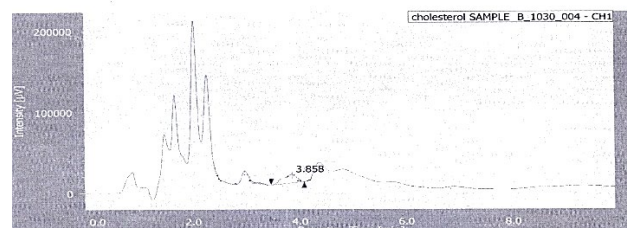
شكل 12: كروماتوجرام عينة لبن البقري منزوع الدسم
