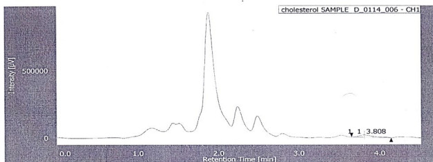
شكل 8: كروماتوجرام عينة ندى منزوع الدسم
