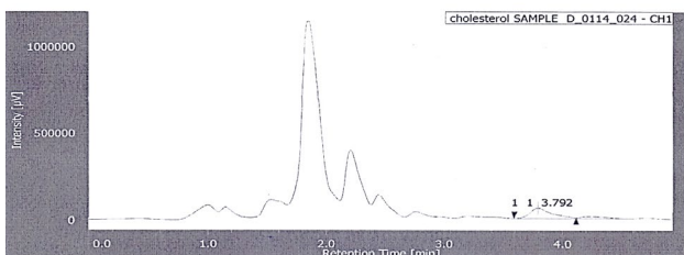
شكل 5: كروماتوجرام عينة لبن الإبل
