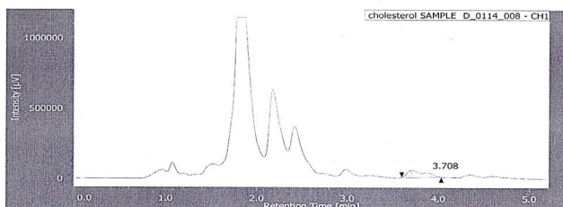
شكل 11: كروماتوجرام عينة لبن يماني
